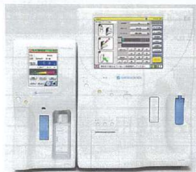
CHM-4100と全自動血球計数器MEK-7300
